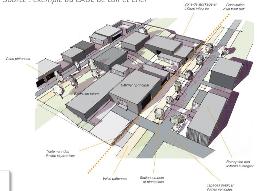
Figure 56 : Implantation et intégration paysagère d'une zone d'activité – Source : exemple du CAUE de Loir et Cher
